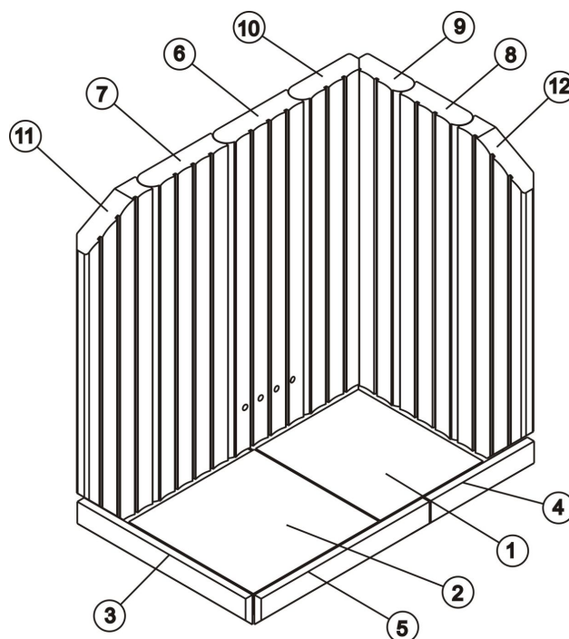
Abb. 1: Zusammenstellung der Schamottesteine Eck-Kamin 45/67/44 STL
